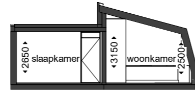
doorsnede bnr. 2.01
