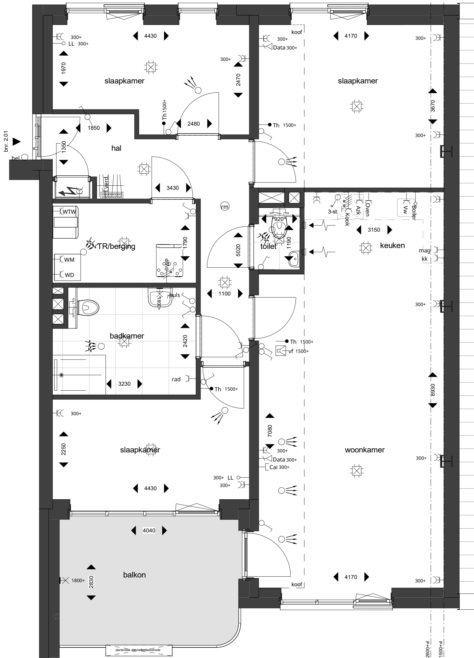
plattegrond bnr. 2.01
